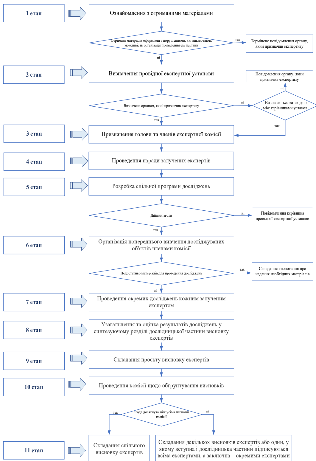
Рис. Алгоритм проведення комплексної судово-медичної експертизи й експертизи зброї
